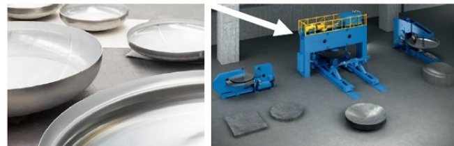
Linhas STD da Relação de Pressas / Manipuladores / Bordeadoras Faccin (R= 42 kg/cm²)
