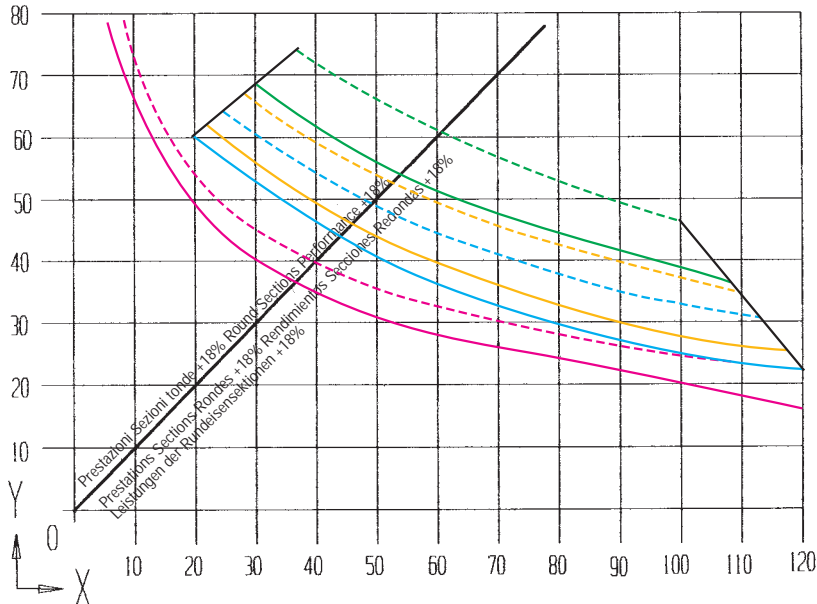
Grafico Prestazioni Profilati in Ferro FE430B - FE430B Iron Section Performance Diagram Grafique Prestations Profils en Fer FE430B - Grafico Rendimientos Perfiles de hierro FE430B Graphik der Leistungen Eisenprofile FE430B
