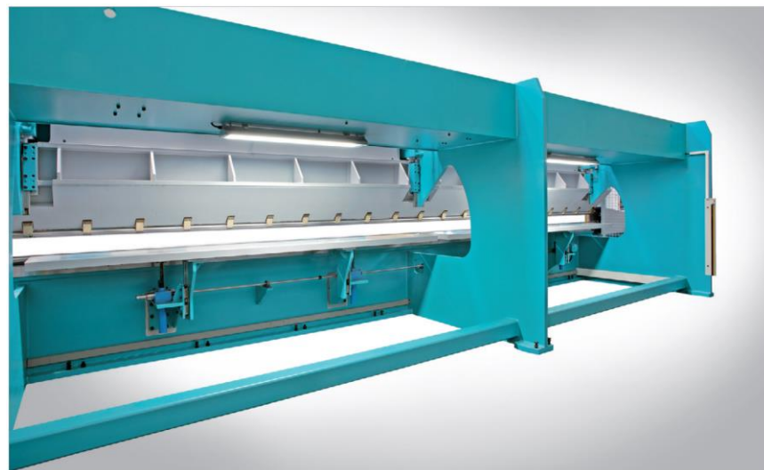
PHC Prensa dobradeira com calandra para a produção de calhas semi-redondas
