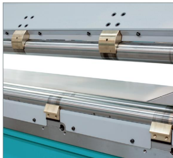
Detalhe dos rolos prensa-calandra com mesa de compensação contínua do rolo superior para evitar possíveis riscos
